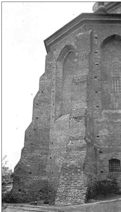
Fot. 6. Mury ceglane z płytkimi otworami maculcowymi (fot. J. Tajchman)
