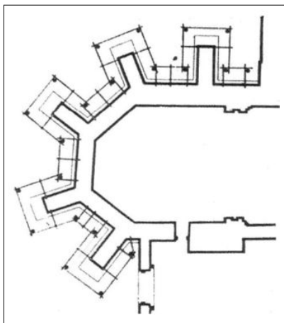
Rys. 16. Szkic rusztowania (szkic ze zbiorów prywatnych prof. B. Guerguina)
